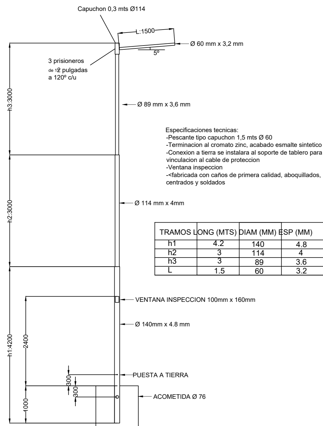
Columna 9m PESCANTE CAPUCHON 1,5m
