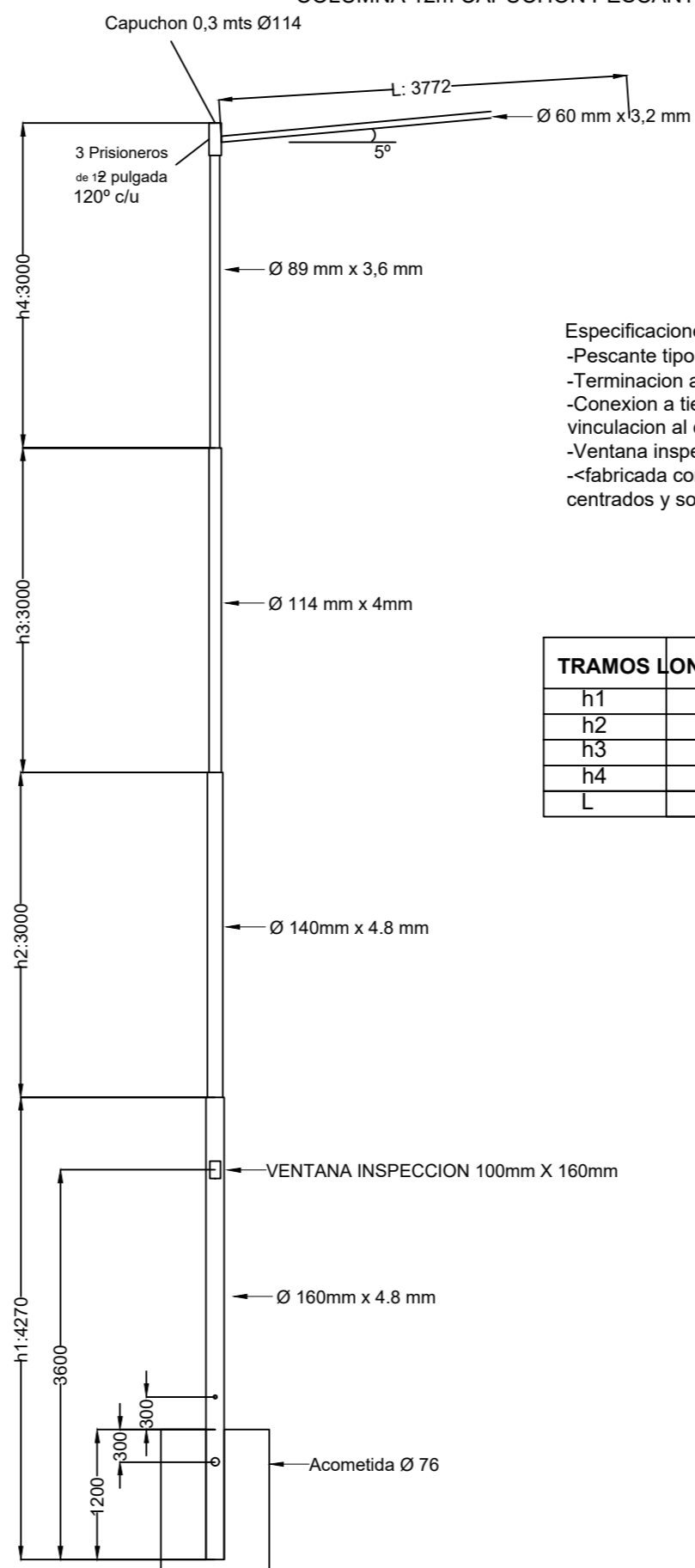
COLUMNA 12m CAPUCHON PESCANTE 2,5mts
