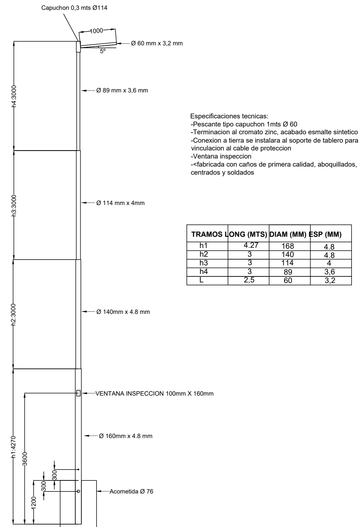
COLUMNA 12m CAPUCHON PESCANTE 1mts
